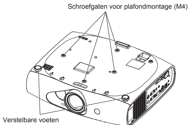
De posities van schroefgaten voor plafondmontage en verstelbare voeten
